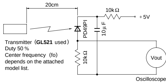
Fig. 1. Transmitter
